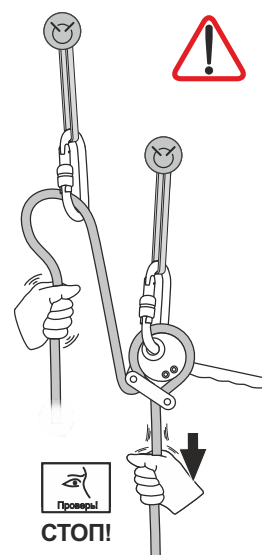
Рис. 12. Простой полиспаст
