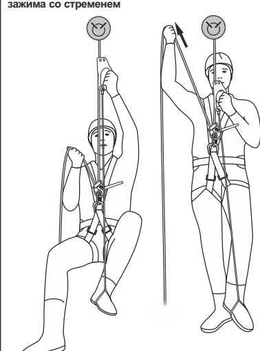
Рис. 11. Подъем с использованием зажима со стремнем
