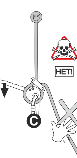
Рис. 10. Контроль каната
