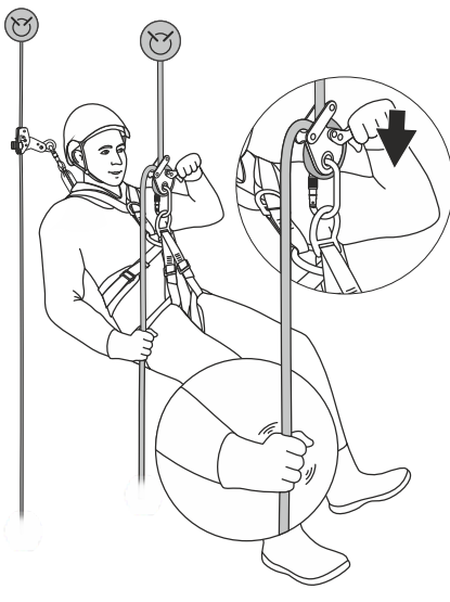
Рис. 10. Контроль каната
