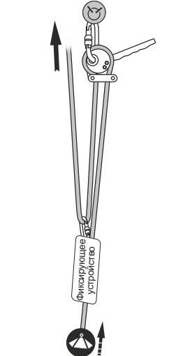
Рис. 12. Простой полиспаст
