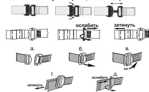
Рис. 6. Типы используемых пряжек, способы заправки
