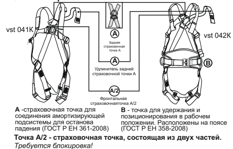
Рис. 3. Маркировка изделия
