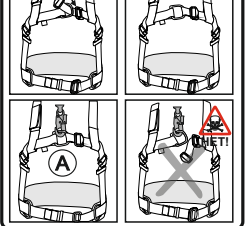
Рис. 12. Способ организации удерживающей системы
