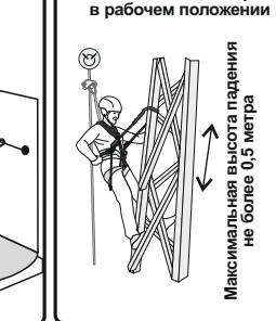
Рис. 13. Позиционирование в рабочем положении
