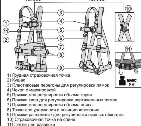
Рис. 2. Типы крепежных точек
