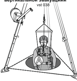
Рис. 13. Способ проведения вертикальной эвакуации vst 038
