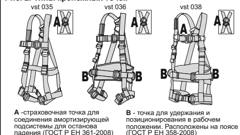
Рис. 2. Типы крепежных точек
