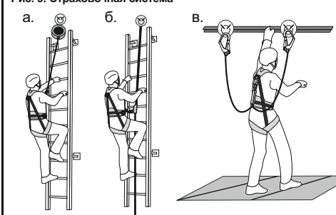
Рис. 9. Страховочная система
