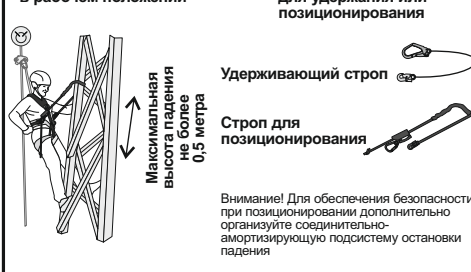
Рис. 12. Позиционирование в рабочем положении
