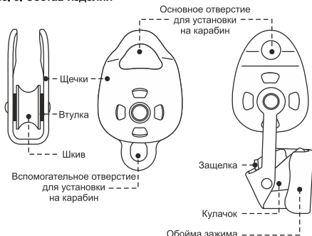
Рис. 3. Состав изделий
