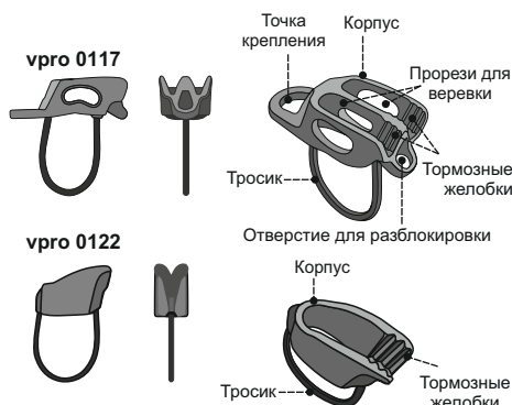
Рис. 1. Общий вид и составные части изделий
