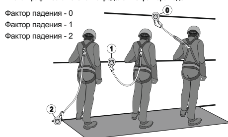
Рис. 3. Графическая схема к определению фактора падения
