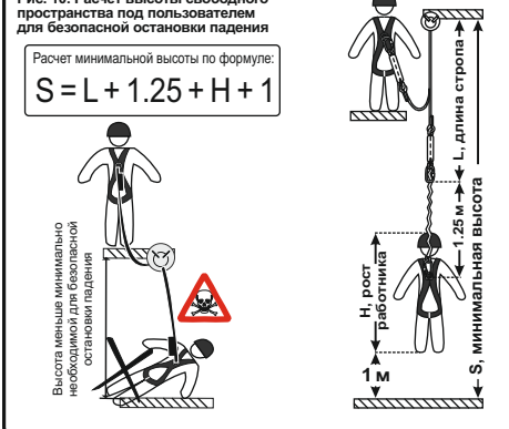
Рис. 10. Расчет высоты свободного пространства под пользователем для безопасной остановки падения
