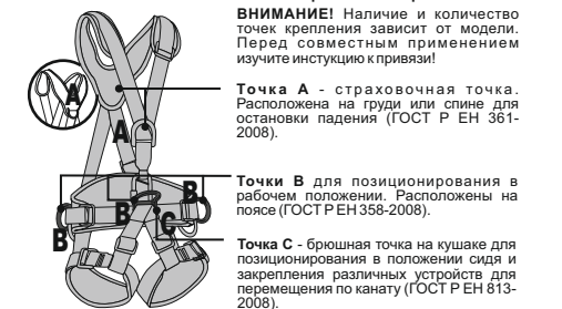
Рис. 4. Расположение и назначение точек крепления на привязях
