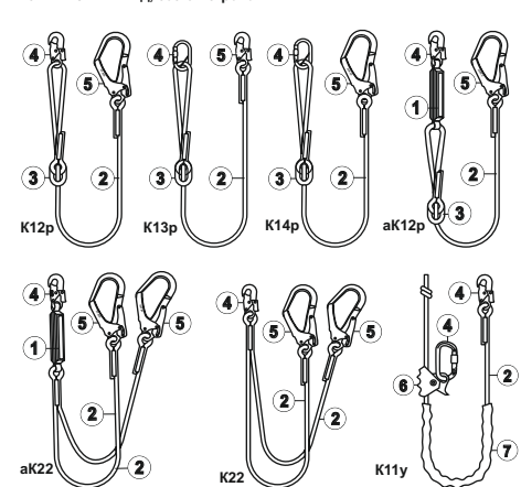
Рис. 1. Внешний вид, состав стропов
