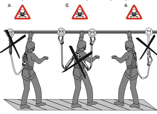
Рис. 11. Ограничения по использованию стропов с амортизатором
