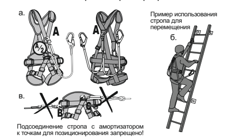
Рис. 5. Использование стропа с амортизатором рывка
