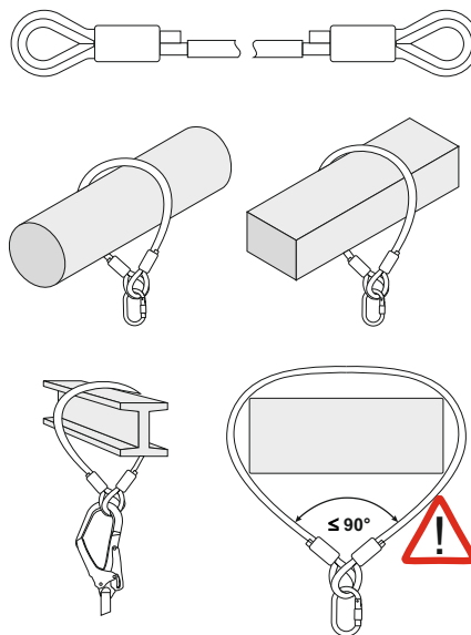
Рис. 3. Установка С10
