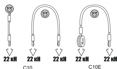
Рис. 5. Допустимое распределение нагрузок
