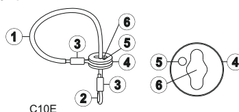
Рис. 4. Установка С10Е
