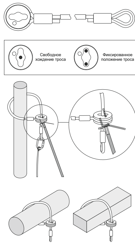
Рис. 4. Установка С10Е
