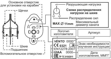
Состав и маркировка блок-роликов (арт.: vрго 0192)
