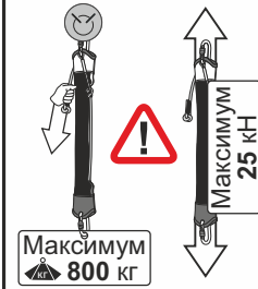
Рис. 9. Допустимые нагрузки
