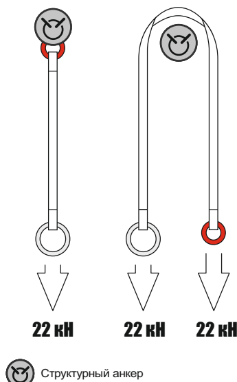
Рис. 3. Допустимое распределение нагрузок
