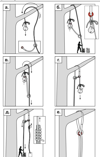
Рис. 4. Способы дистанционной инсталляции к анкерному устройству
