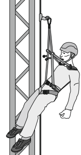
Рис. 12. Срабатывание страховочной системы
