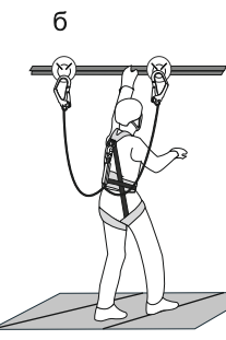
Рис. 11. Страховочная система
