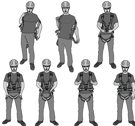
Рис. 6. Надевание привязи «Энерго»
