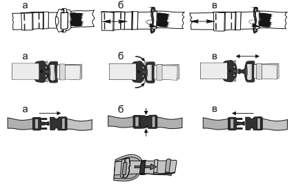
Рис. 7. Натяжение лямок
