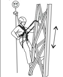
Рис. 14. Позиционирование в рабочем положении
