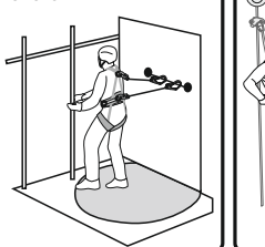
Рис. 15. Пример организации системы канатного доступа
