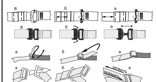
Рис. 5. Типы используемых пряжек, способы заправки
