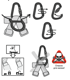
Рис. 10. Страховочная система
