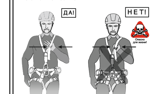
Рис. 11. Соединительно-амортизирующая подсистема
