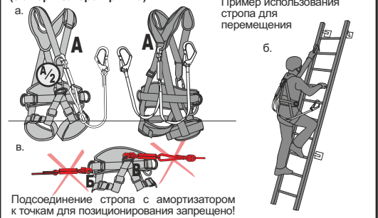
Рис. 8. Ограничения по использованию стропов с амортизатором
